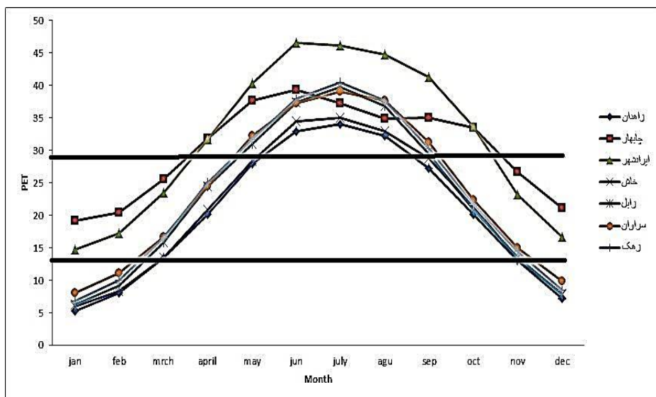
شکل ۲: تغییرات شاخص دمای معادل فیزیولوژیک در ایستگاه‌های سینوپتیک منطقه جنوب شرق
