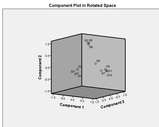
شکل ۲: نمودار سه‌بعدی پراکنش متغیرها نسبت به عامل‌های استخراج‌شده
